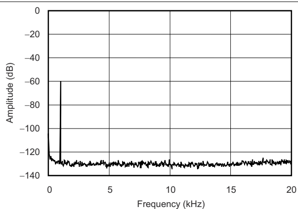
FIG 6-10. Output Spectrum
