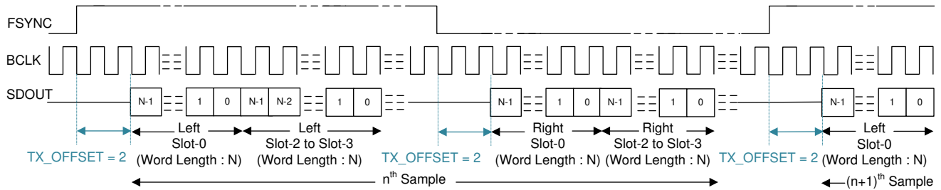
7-10. LJ Protocol Timing (TX_OFFSET = 2)
