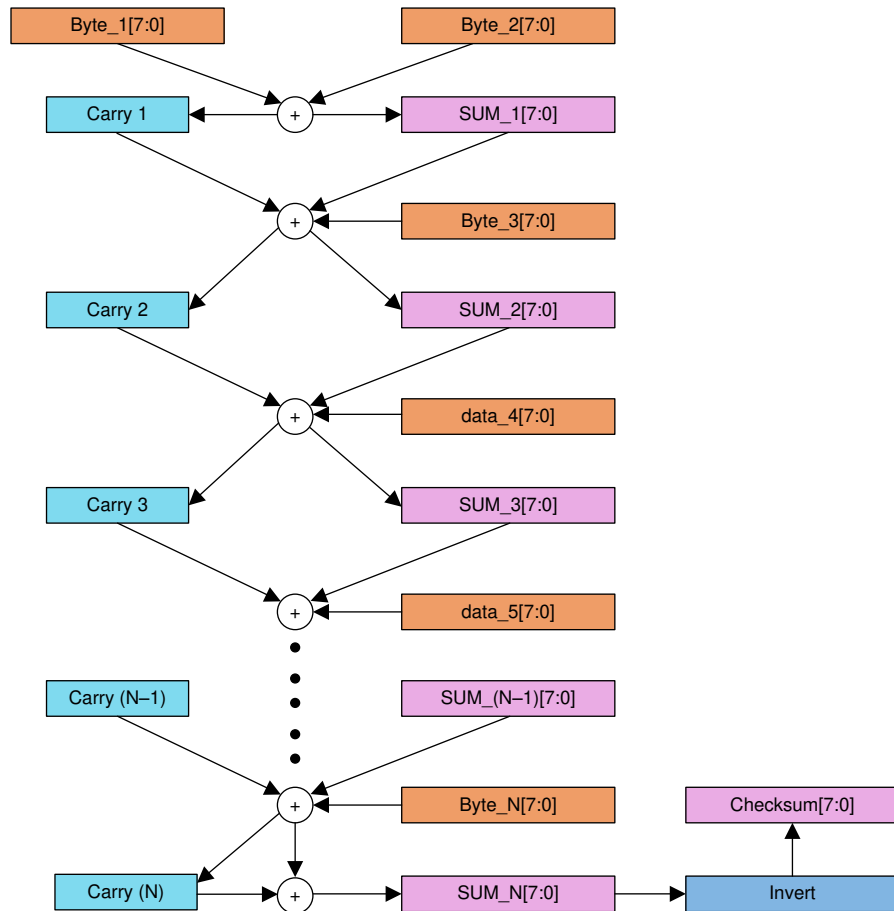
図 7-17. チェックサム計算
