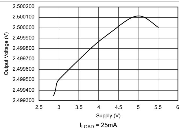
図 6-40. 出力電圧対電源電圧 I_{LOAD} = 25\text{mA}
