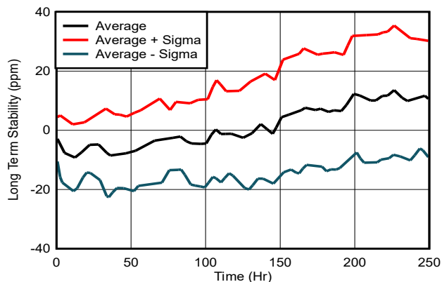
図 6-22. 長期安定性: 0~250 時間
