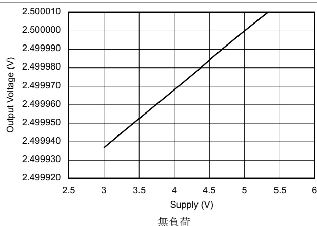
図 6-39. 出力電圧対電源電圧 無負荷
