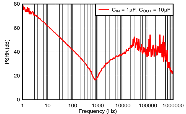
図 6-16. 電源除去比と周波数との関係
