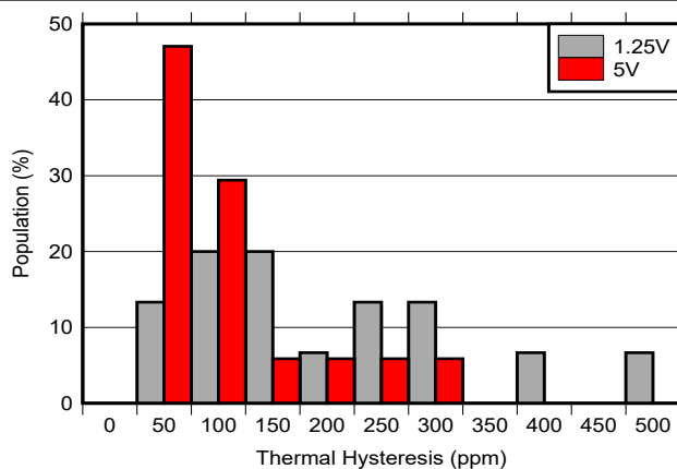
図 6-24. 熱ヒステリシス ヒストグラム (-40°C ~ 125°C、サイクル 1)
