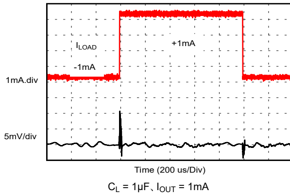
図 6-17. 負荷過渡
