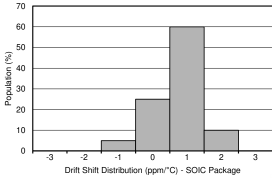
図 7-9. ドリフトのシフトの分散、SOIC パッケージ
