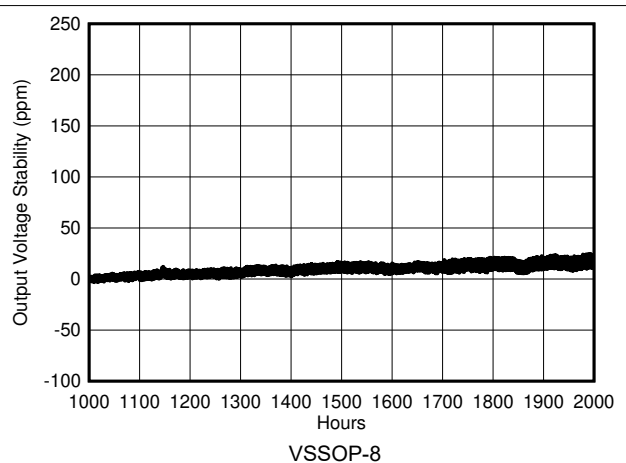
図 6-24. REF50xx の長期安定性 (2 番目の 1000 時間)
