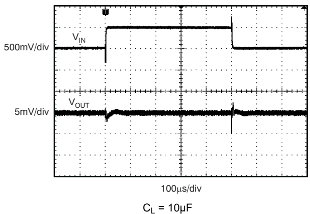
図 6-22. ライン トランジェント
