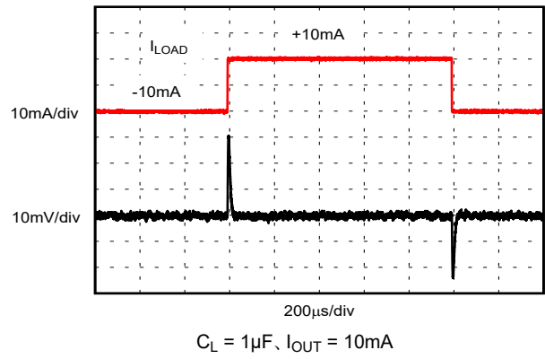
図 6-18. 負荷過渡
