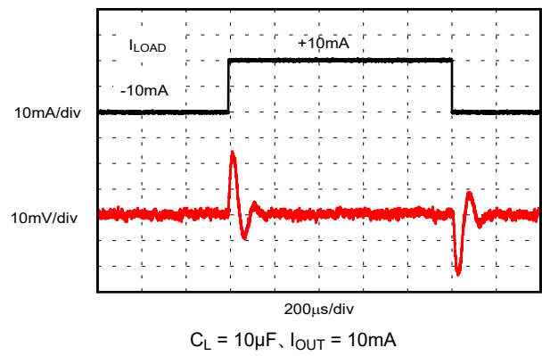
図 6-20. 負荷過渡
