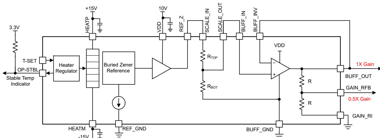
REF81 のブロック図 (代表的な外部接続を含む)
