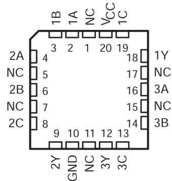
図 4-2. SN54AC10 FK パッケージ (上面図)
