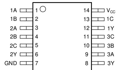
図 4-4. SN74AC10 D、DB、N、NS、PW パッケージ (上面図)
