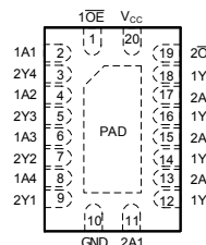
図 4-4. SN74ACT244: RKS Packages, 20-Pin VQFN (Top View)
