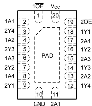
図 4-4. SN74AHC244 RKS パッケージ、20 ピン VQFN (上面図)
