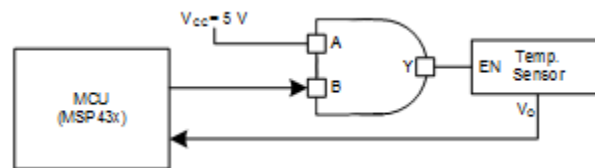
図 7-1. 電源シーケンス アプリケーション
