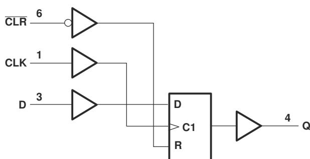
ロジック図
