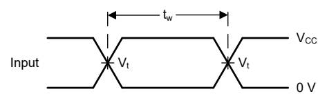
図 6-2. 電圧波形、パルス幅
