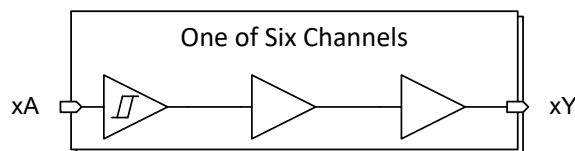
概略ロジック図
