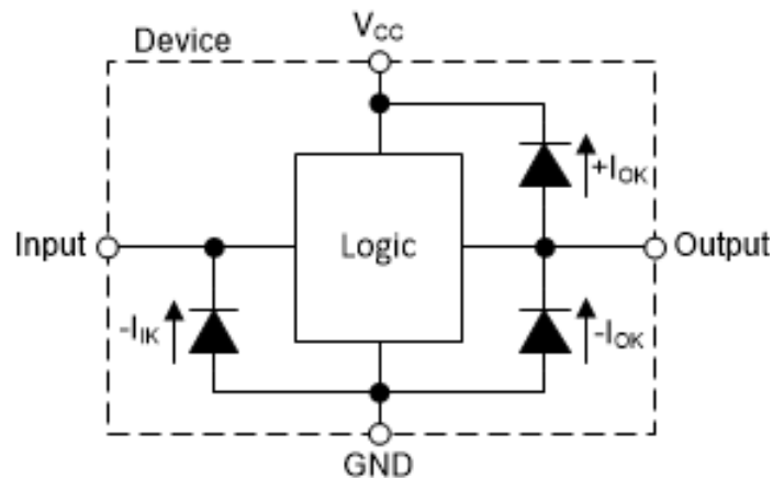
図 6-3. 各入力と出力に対するクランプ ダイオードの電気的配置
