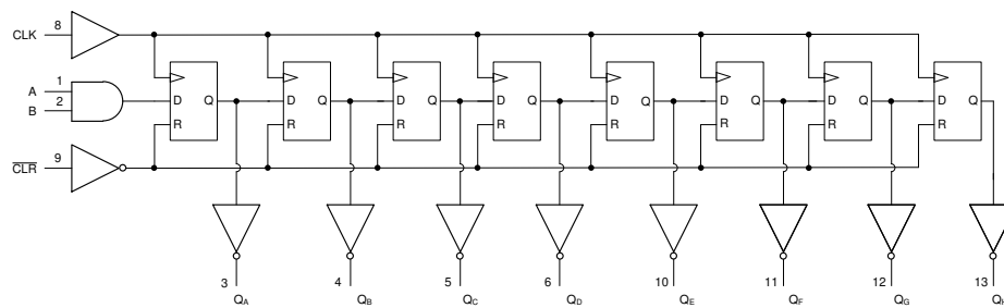
論理図 (正論理)
