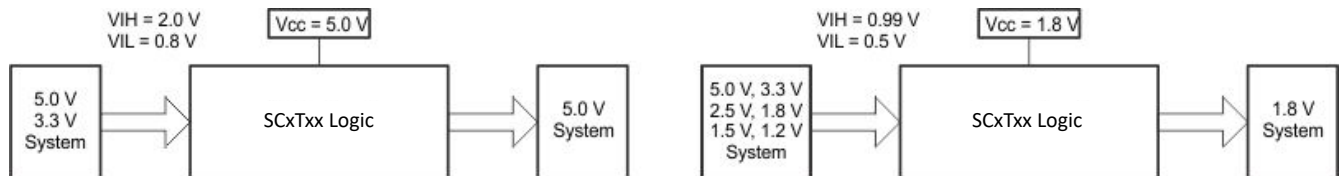
図 6-2. SCxT の昇圧および降圧変換の例
