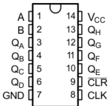
図 4-1. PW パッケージ 14 ピン TSSOP (上面図)
