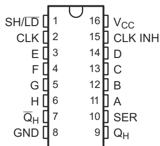
図 4-1. PW パッケージ、 16 ピン TSSOP (上面図)
