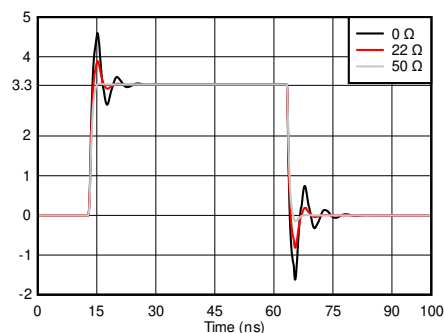
図 8-2. スイッチング特性の比較
