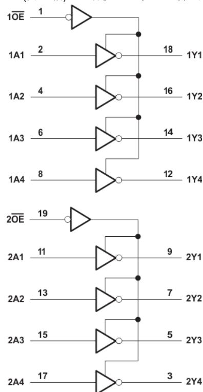
論理図 (正論理)
