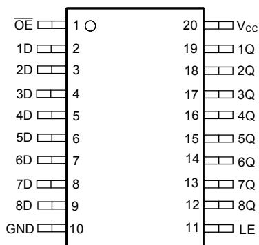
PW パッケージ (上面図)
