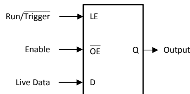
図 8-1. 代表的なアプリケーション回路図
