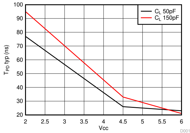
図 8-2. 伝搬遅延時間曲線 (標準値)
