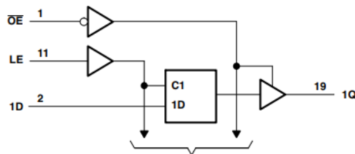
図 7-1. 論理図 (正論理)
