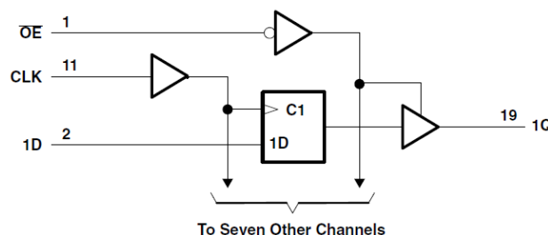
論理図 (正論理)
