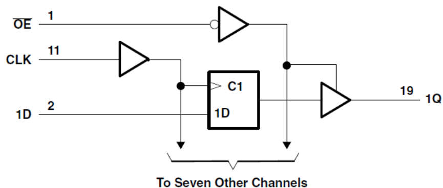
図 7-4. 論理図 (正論理)
