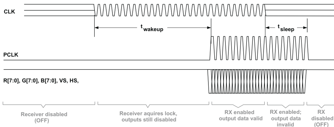
图 7-11. Standby Detection
