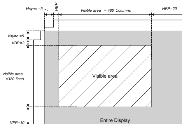
图 9-1. HVGA Display
