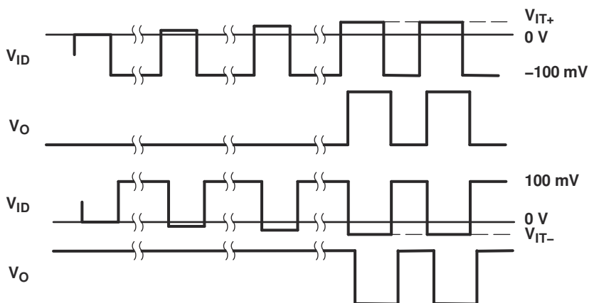
図 7-4. V_{IT+} および V_{IT-} 入力電圧スレッシュホルドのテスト回路と定義
