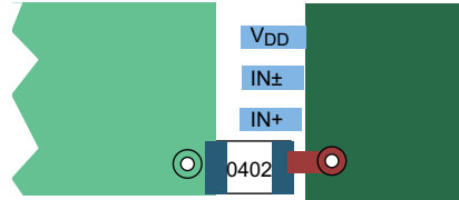
図 11-8. デカップリング コンデンサの標準レイアウト (b)
