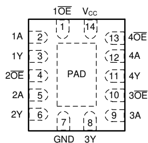
図 4-1. SN74AC126-Q1 BQA または パッケージ (上面図)
