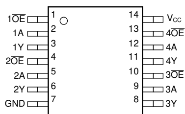
図 4-2. SN74AC126-Q1、PW パッケージ (上面図)
