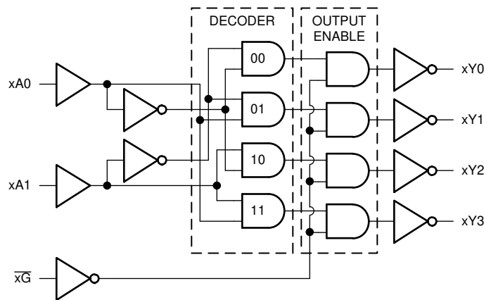
図 7-1. SN74AC139-Q1 -Q1 の論理図 (正論理)
