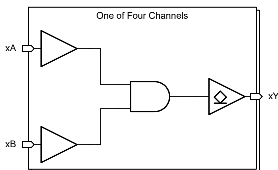
機能ブロック図
