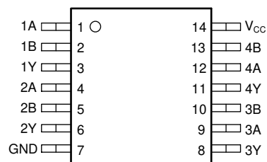
図 4-2. SN74ACT09、PW パッケージ (上面図)
