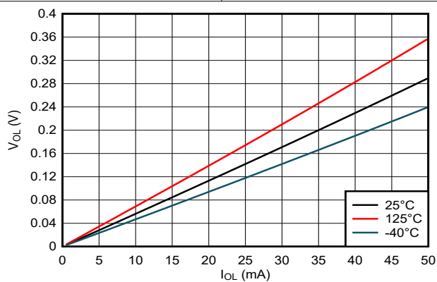
図 5-4. Low 状態における出力電圧と電流との関係、5V 電源
