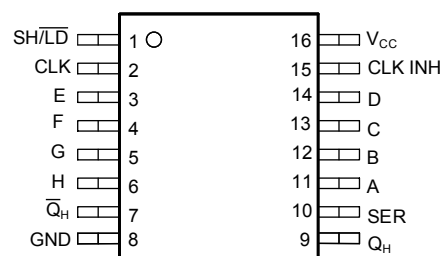
図 4-2. SN74ACT165 PW パッケージ (上面図)
