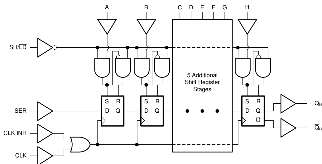
図 7-1. SN74ACT165 の論理図 (正論理)
