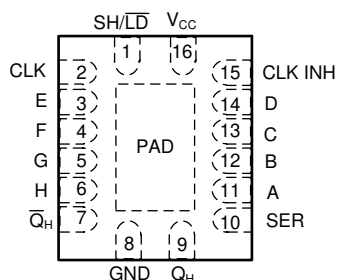
図 4-1. SN74ACT165 BQB パッケージ (上面図)
