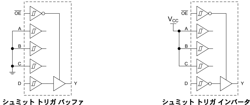
図 7-1. ロジック構成
