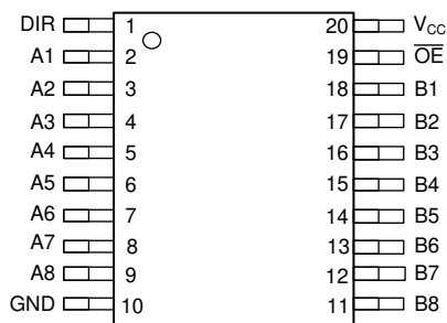
図 4-1. SN74AHC245-Q1 PW または DGS パッケージ、20 ピン TSSOP または VSSOP (上面図)
