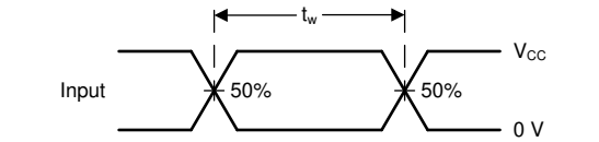
図 6-2. 電圧波形、パルス幅
