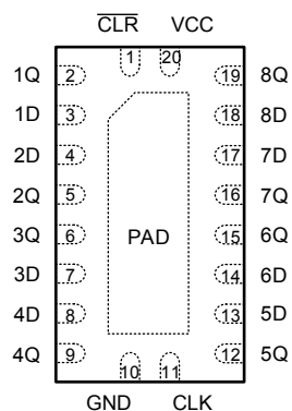
図 4-1. SN74AHC273-Q1 RKS または RGY パッケージ (上面図)
