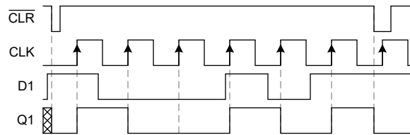
図 8-2. 「アプリケーションのタイミング図」、1 つのデータ チャネルを示します
