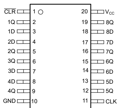
図 4-2. SN74AHC273-Q1 PW、DGS パッケージ (上面図)
