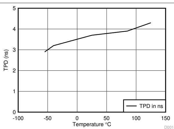
図 5-2. TPD vs Temperature
