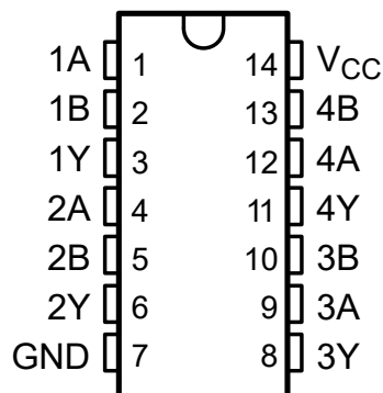
図 4-1. D または PW パッケージ、14 ピン SOIC または TSSOP (上面図)
