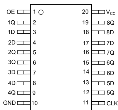
図 4-1. SN74AHCT374-Q1 RKS パッケージ (上面図) 図 4-2. SN74AHCT374-Q1 PW、DGS パッケージ (上面図)
