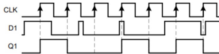
図 7-2. クロック動作を示す概略機能図
