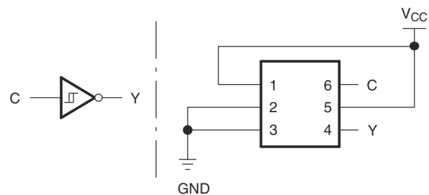
图 7-9. 04/14: Inverter
