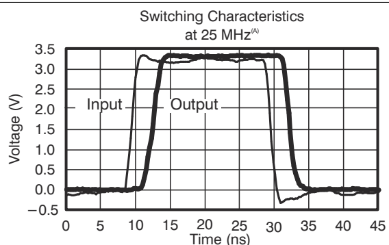
図 5-2. 優れたシグナル インテグリティ
