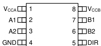
図 4-1. DCT パッケージ、8 ピン SSOP (上面図)
