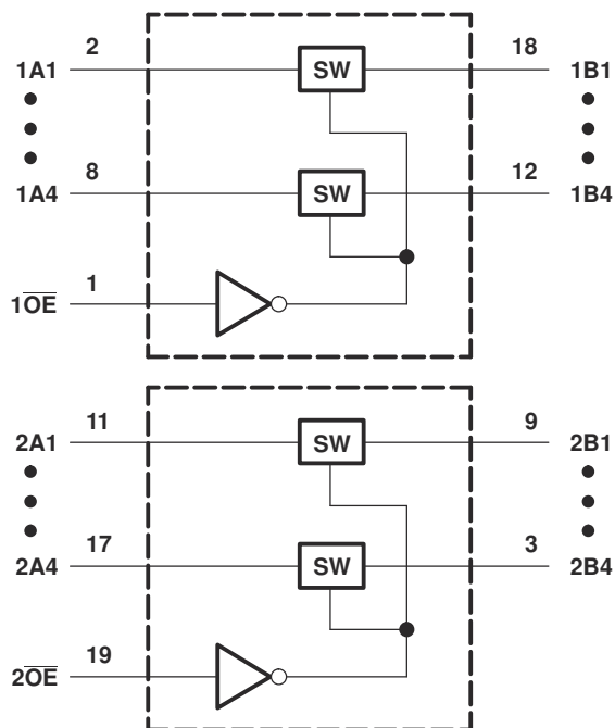
論理図 (正論理)
