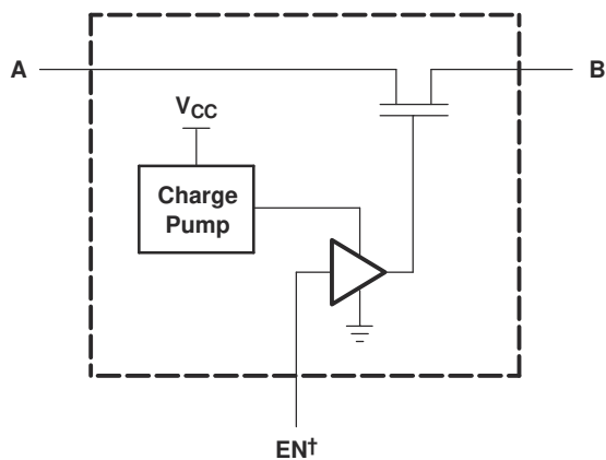
論理図 (正論理)
