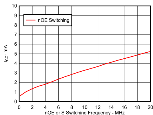
図 4-2. 標準値 I_{CC} と \overline{OE} のスイッチング周波数
