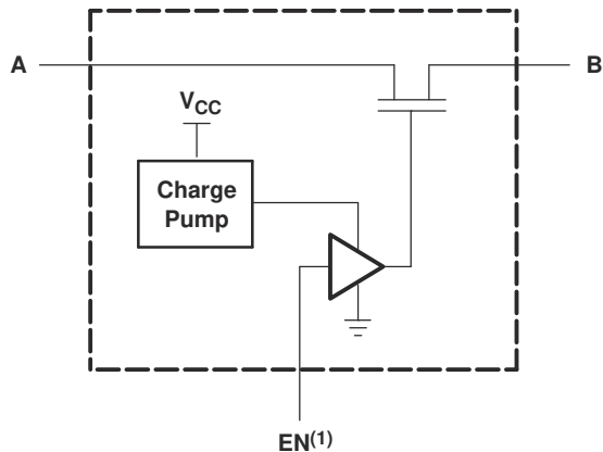
図 3-3. 概略回路図、各 FET スイッチ (SW)
