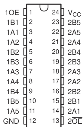
図 3-1. ピン配置
