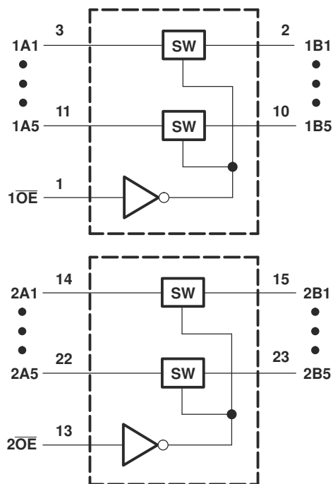
図 3-2. 論理図 (正論理)
