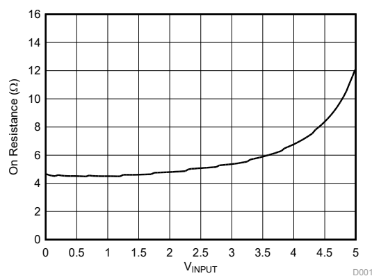
図 4-1. 標準値 r_{on} と V_I
