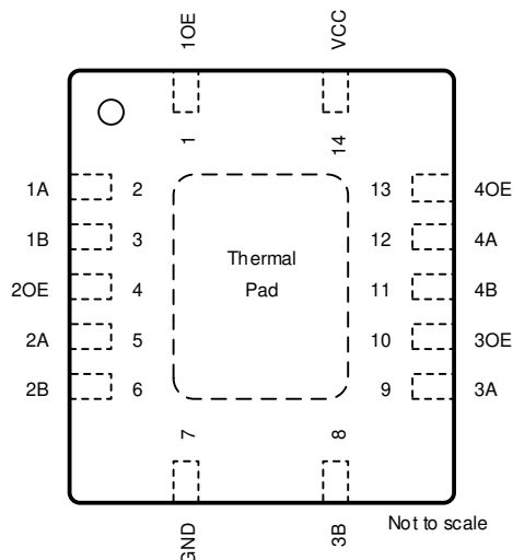
図 4-2. BQA パッケージ、14 ピン WQFN (上面図)
