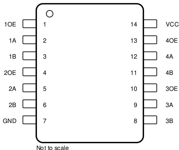
図 4-1. PW および DYY パッケージ、14 ピン TSSOP および SOT (上面図)
