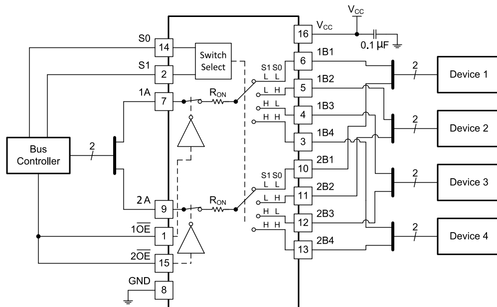
図 8-1. SN74CBTLV3253-Q1 の代表的なアプリケーション
