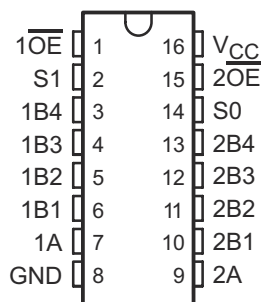
図 4-1. PW または DYY パッケージ 16 ピン TSSOP または SOT 上面図
