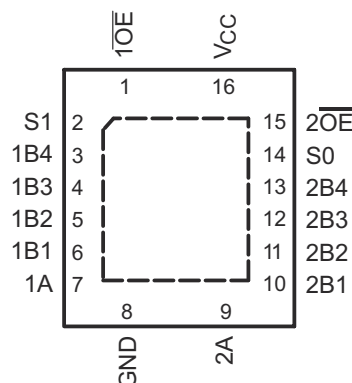
図 4-2. BQB パッケージ 16 ピン VQFN 上面図
