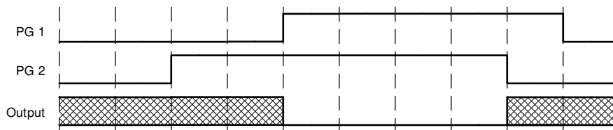
図 8-2. アプリケーションのタイミング図
