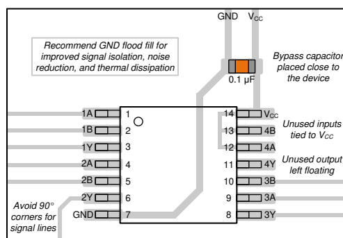
図 8-3. SN74HCS03 のレイアウト例
