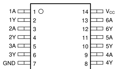
図 4-1. PW、D、または DYY パッケージ、14 ピン TSSOP、SOIC、または SOT-23 上面図
