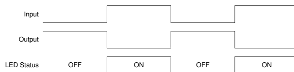
図 8-2. アプリケーションのタイミング図
