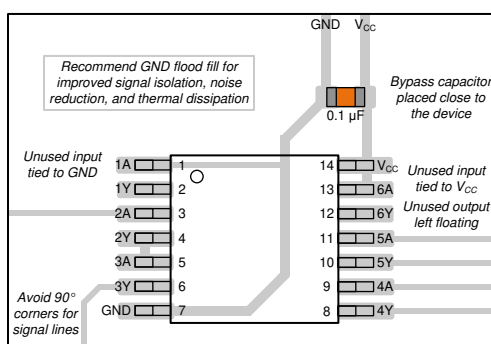
図 8-3. SN74HCS05 のレイアウト例
