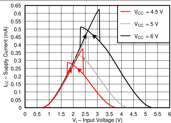
図 5-3. 一般的な電源値 (4.5V ~ 6V) における標準的な電源電流と入力電圧との関係
