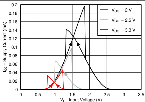
図 5-2. 一般的な電源値 (2V ~ 3.3V) における標準的な電源電流と入力電圧との関係
