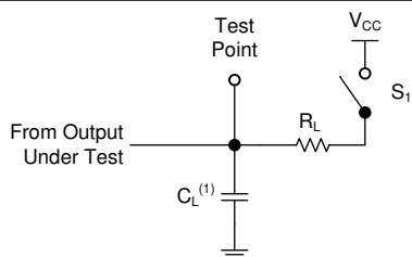
図 6-1. 負荷回路
