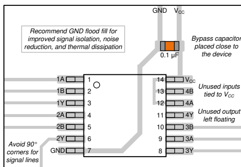
図 8-3. SN74HCS09 のレイアウト例
