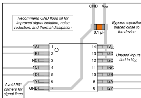
図 8-3. SN74HCS20 のレイアウト例
