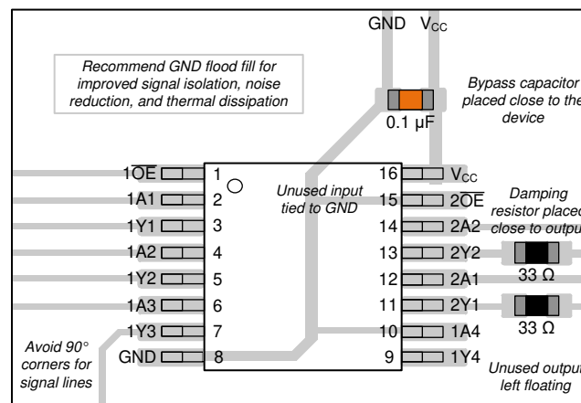
図 8-3. PW パッケージに封止した SN74HCS367 のレイアウト例
