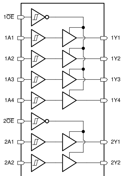
図 7-1. SN74HCS367 の論理図 (正論理)
