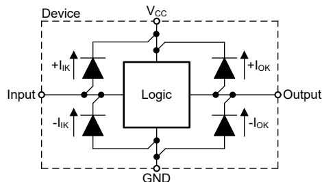
図 7-2. 各入力と出力に対するクランプ ダイオードの電気的配置
