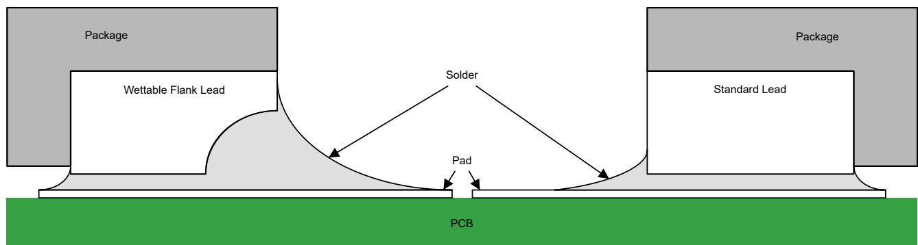
図 7-3. 半田付け後のウェットابل フランク QFN パッケージと標準 QFN パッケージの概略断面図
