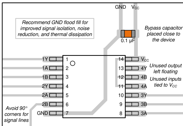
図 8-3. レイアウト例：SN74LV4T02-EP
