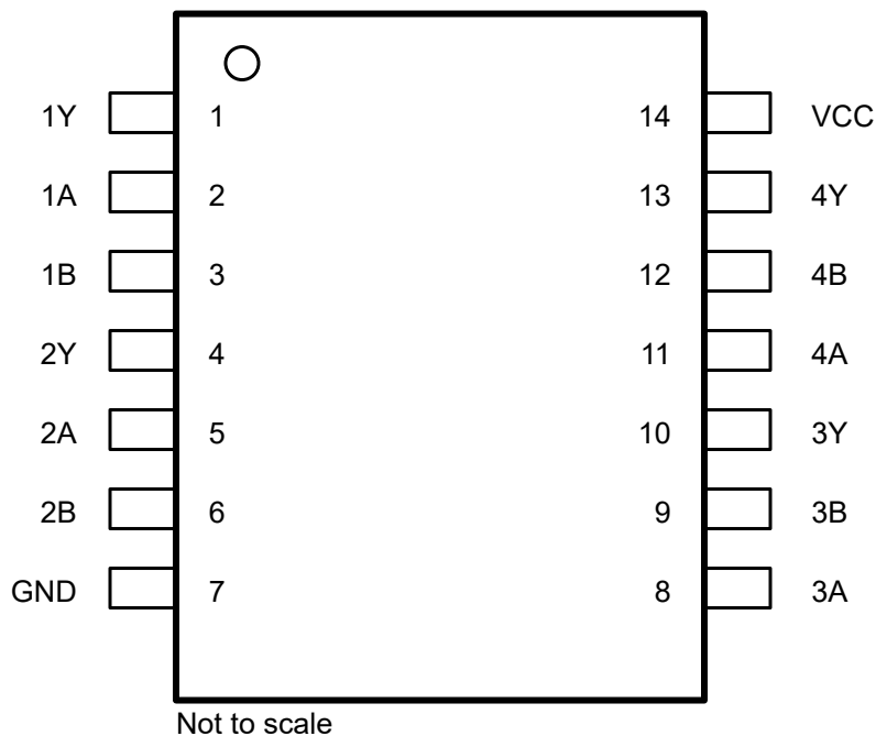
図 4-1. PW パッケージ、14 ピン TSSOP (上面図)
