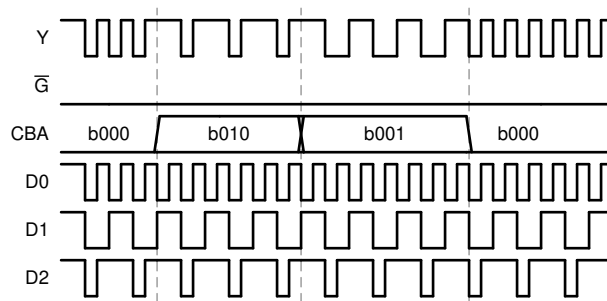
図 8-2. アプリケーション タイミング図
