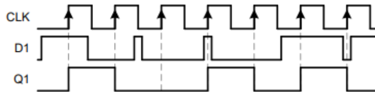
図 9-2. クロック動作を示す概略機能図
