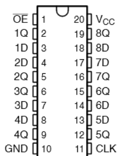
図 7-1. PW パッケージ 20 ピン TSSOP (上面図)
