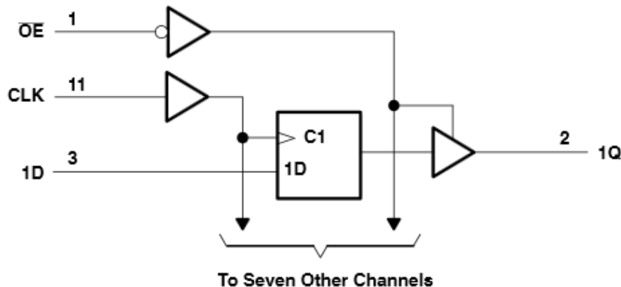
図 8-1. 論理図 (正論理)
