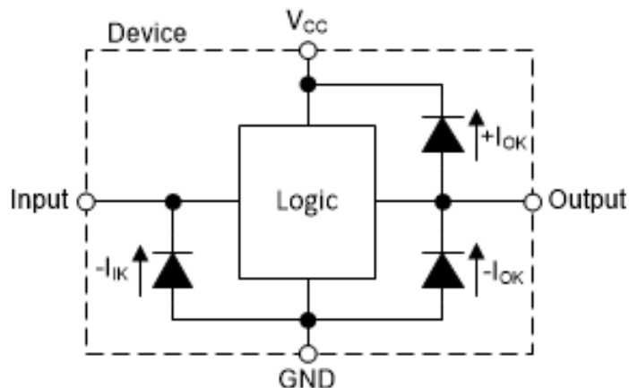
図 8-4. 各入力と出力に対するクランプ ダイオードの電氣的配置
