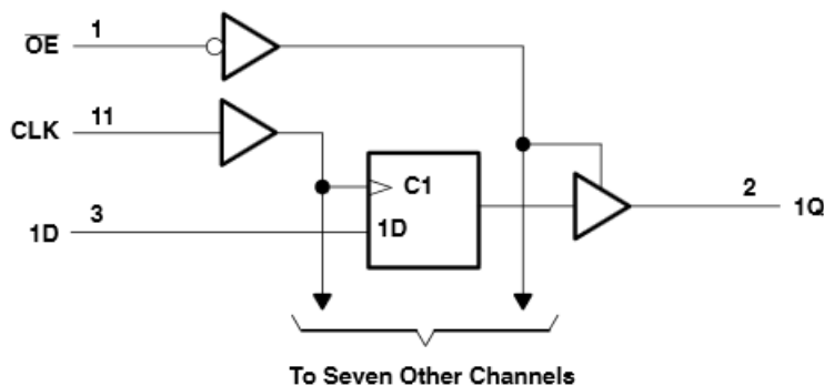
論理図 (正論理)
