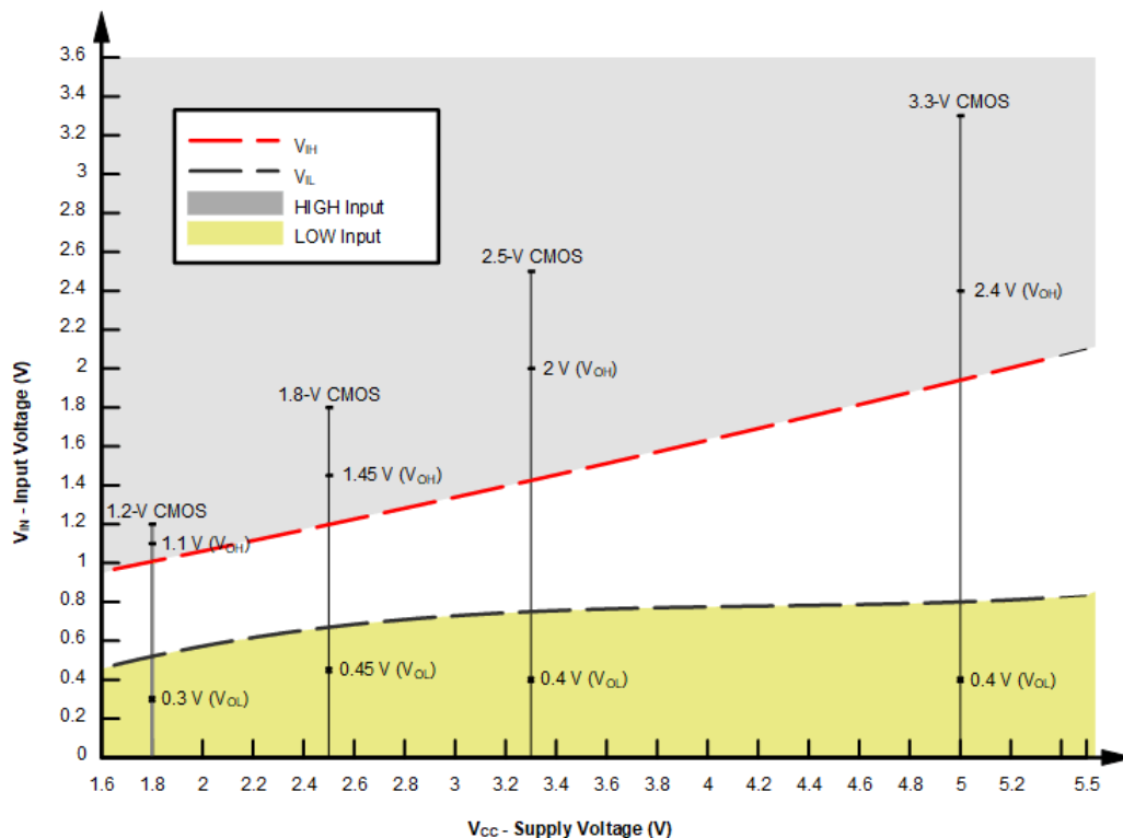
図 7-1. LVxT の 電圧レベル
