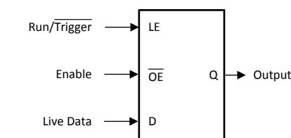
図 8-1. 代表的なアプリケーション回路図
