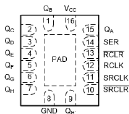
図 4-2. BQB パッケージ、16 ピン WQFN (透過上面図)
