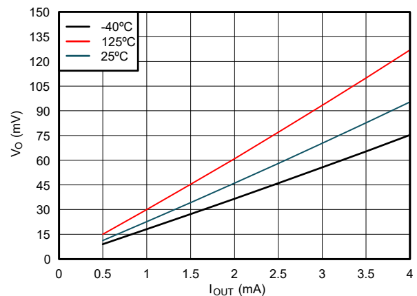
図 5-5. Low 状態における出力電圧と電流との関係、1.65V 電源
