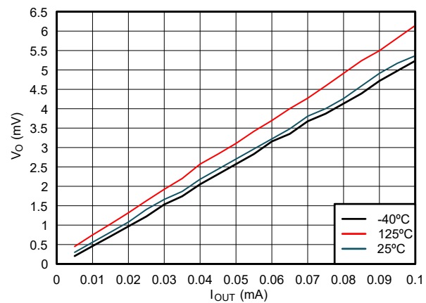
図 5-7. Low 状態における出力電圧と電流との関係、1.1V 電源
