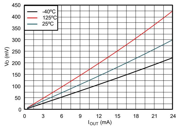
図 5-3. Low 状態における出力電圧と電流との関係、3V 電源
