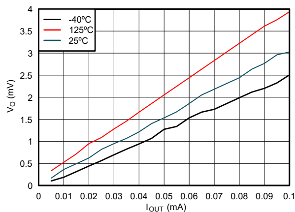
図 5-6. Low 状態における出力電圧と電流との関係、1.38V 電源
