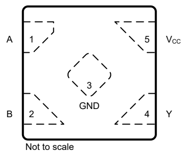
図 4-2. DTX パッケージ、 5 ピン X2SON（上面図）
