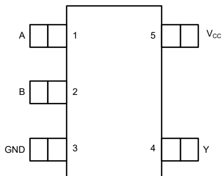
図 4-1. DBV または DCK パッケージ、 5 ピン SOT-23 または SOT-SC70（上面図）
